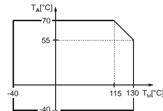
Temperaturgrenzen der AC-Ausführungen, [T A ] Umgebungstemperatur [T M ] Medientemperatur
