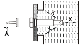
Flanschausführung, kritische Abstände: x > 5\text{mm}
