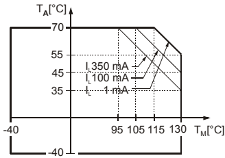
Temperaturgrenzen der DC-Ausführungen, [I_L] Laststrom
