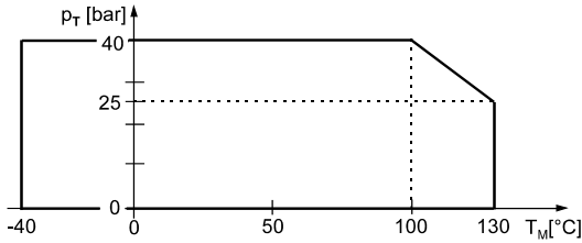
Druck [p_T] in Abhängigkeit von Temperatur [T_M] für alle Ausführungen (außer PP-Flasch-Ausführung)
