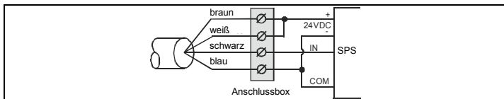
Unterer Grenzwertschaltpunkt
