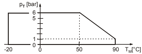
Druck [p_T] in Abhängigkeit von Temperatur [T_M] für PP-Flasch-Ausführung
