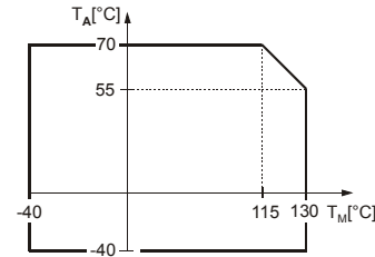
Temperaturgrenzen der AC-Ausführungen, [T_A] Umgebungstemperatur [T_M] Medientemperatur
