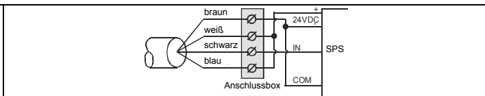
Oberer Grenzwertschaltpunkt
