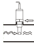
Flanschausführung, kritische Abstände: x > 5\text{mm}
