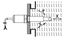
Flanschausführung, kritische Abstände: x > 5\text{mm}
