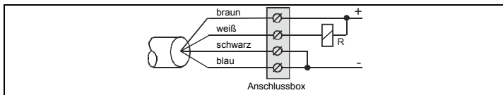
Unterer Grenzwertschaltpunkt
