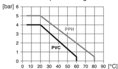
Druck-Temperatur Diagramm
